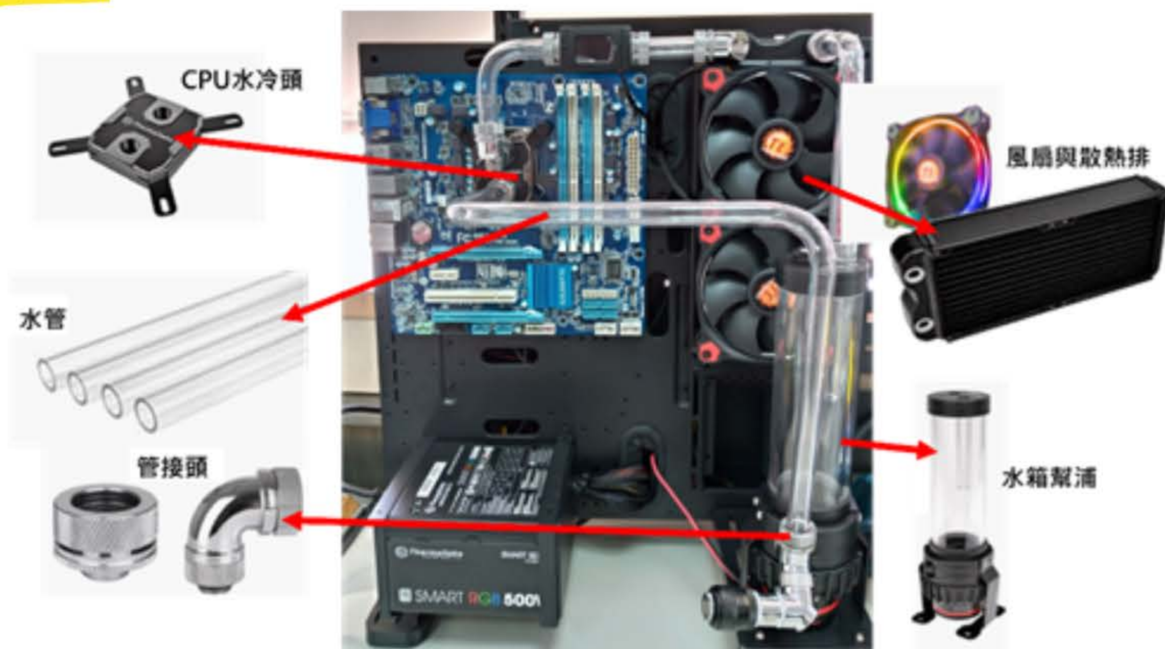
圖一 競賽水冷電腦主機參考圖
