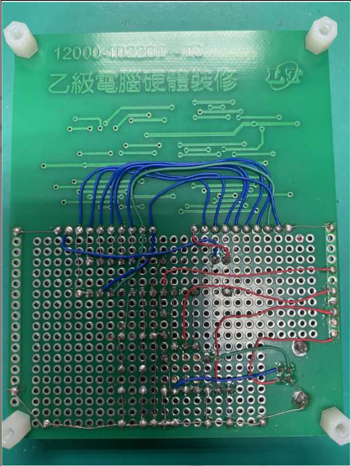
電路板
